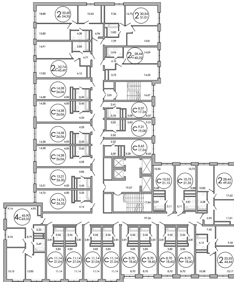
План этажа
