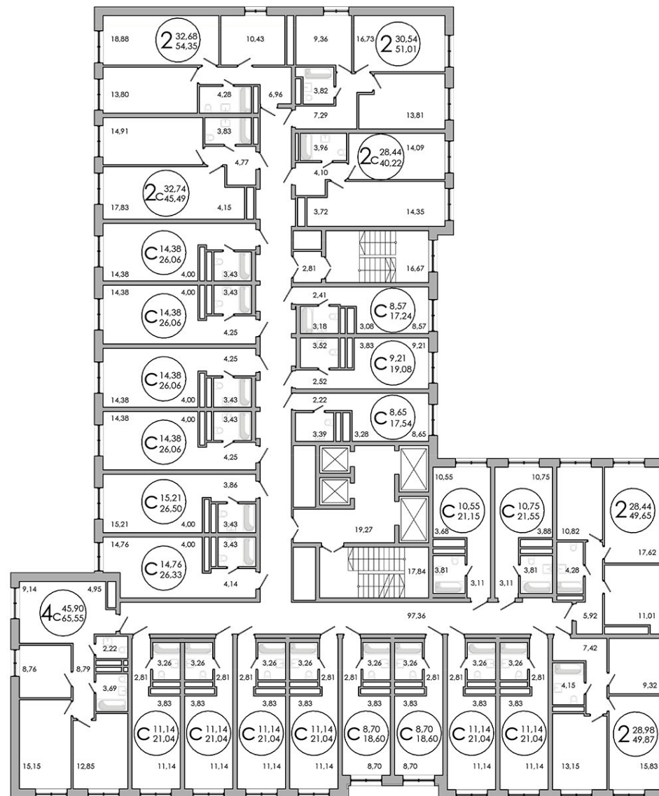
План этажа
